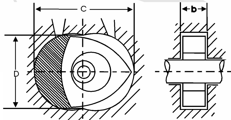
Berechnung der Verdrängung eines Kreiskolbenmotors
